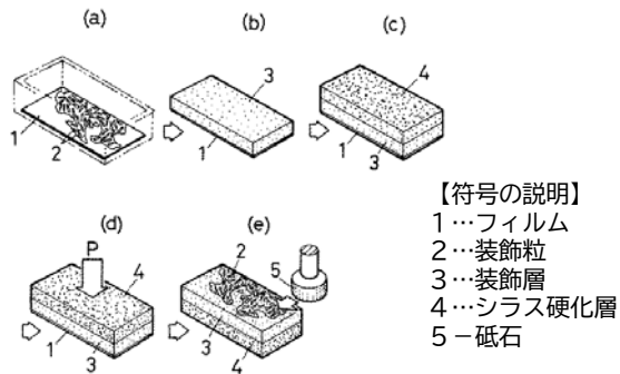
シラスコンクリート装飾板の製造方法工程図
