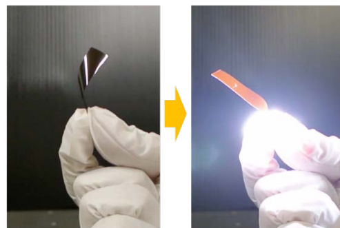
図1. 光を浴びて変形するアモルファス窒化炭素薄膜
